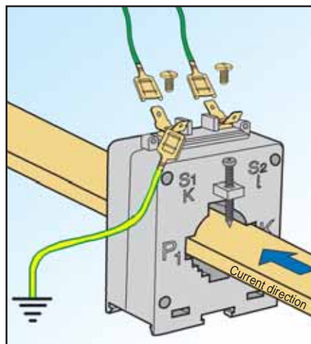
AVEC FASTON (6,3 mm)
