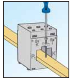
CABLAGE SUR BUS BARRE
