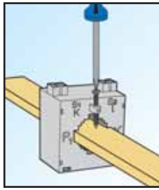
CABLAGE SUR BUS BARRE
