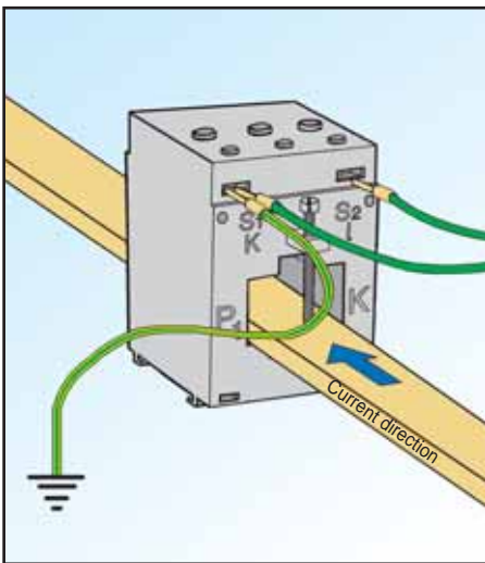
AVEC EMBOUT MÉTALLIQUE
