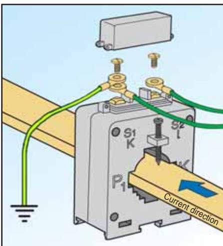
AVEC COSSE RONDE
