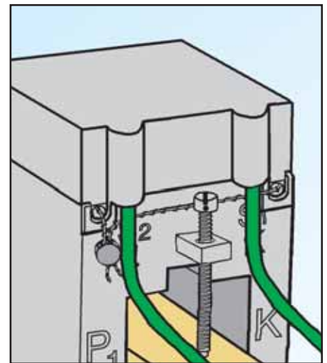
MONTAGE DU CAPOT DE PROTECTION ET SELLAGE
