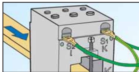
AVEC FASTON (6,3 mm)
